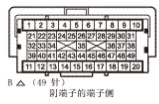
PCM 连接器端子位置
